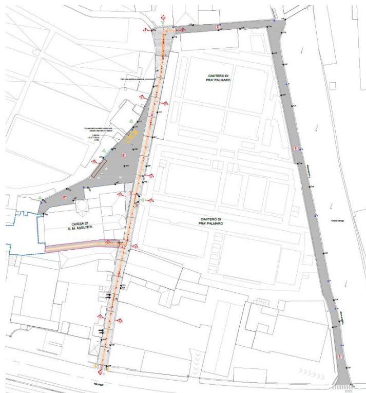
Planimetria dell'intervento
